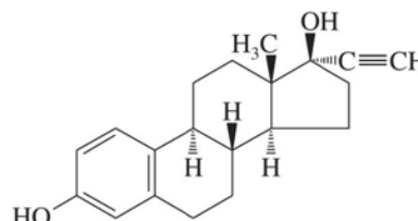
Ethinyl estradiol [17 \alpha -ethynyl-1,3,5(10)-estratriene-3,17 \beta -diol]
