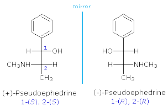
Pseudoephedrine enantiomers
