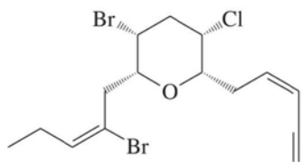
Dactylene
