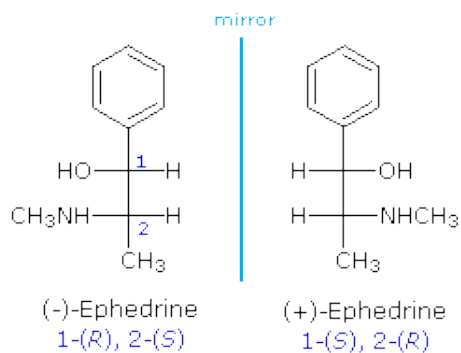
Ephedrine enantiomers
